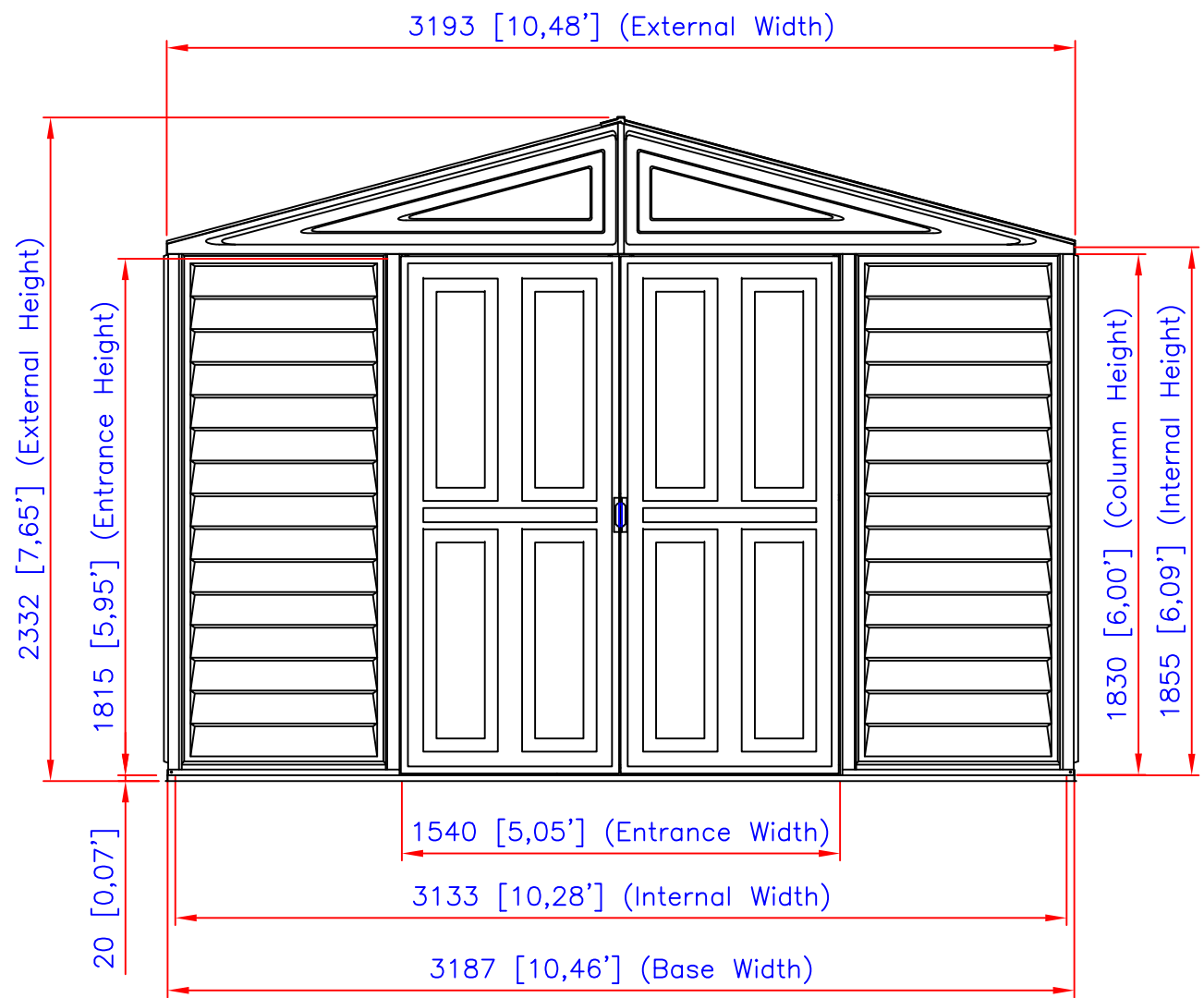
Elevation
